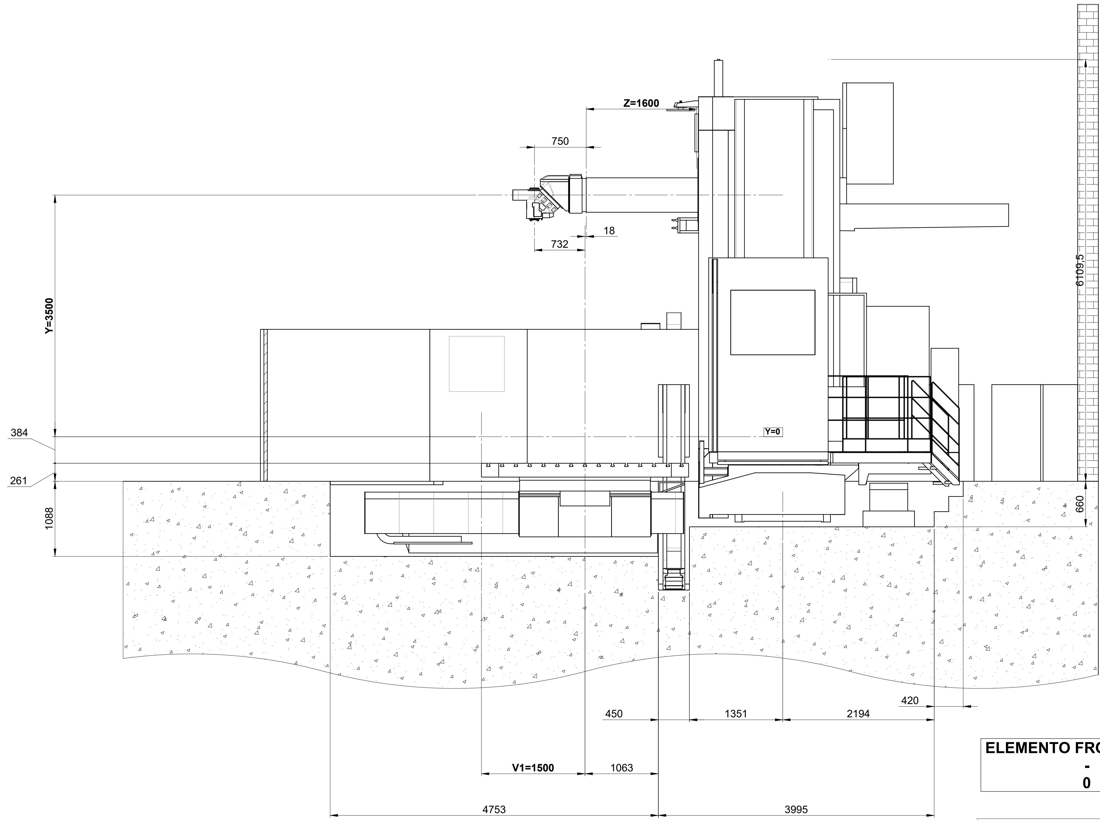
B-B 270°
